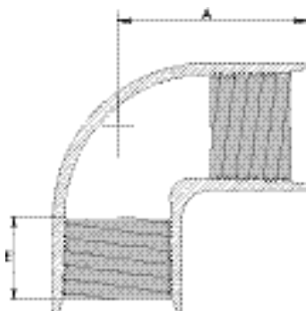
CODO 90°
